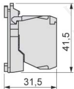
ZB5-AZ104
