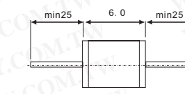
2R-A 2 L TYPE (Φ5.5×6)
