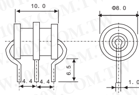
3R-AL, TYPE (Φ8×10)
