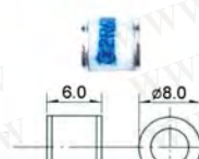
2R-As Type (Φ8×6)
