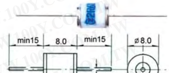
2R-AsL Type (Φ8×8)
