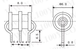
3R-AL, TYPE (Φ6×8)
